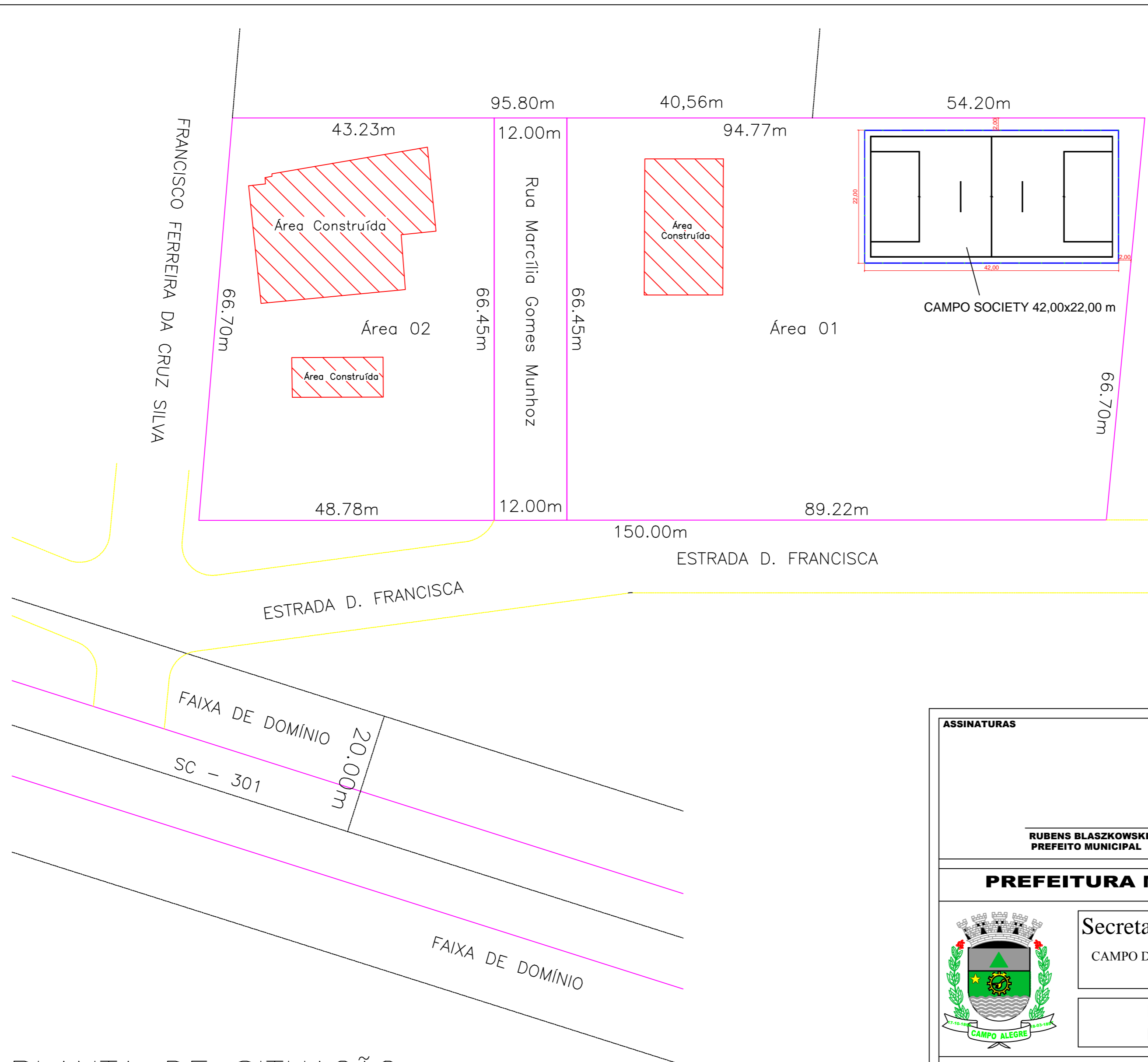
PLANTA DE SITUAÇÃO ESC.: 1:500
